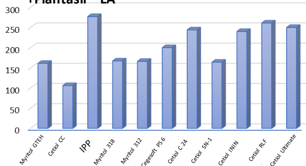
Datos de viscosidad de diferentes aceites +Plantasil® LA
